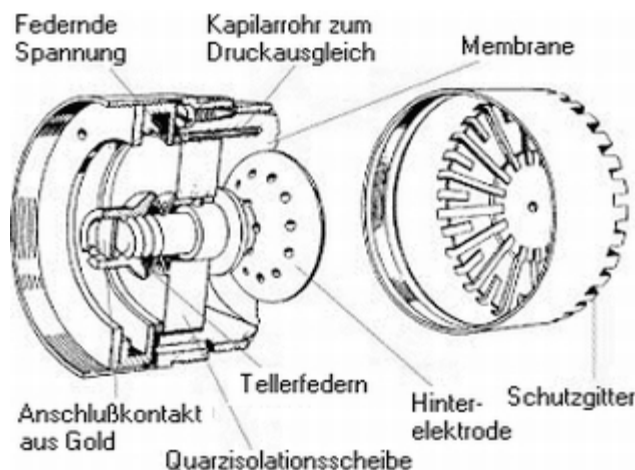
Abb. 13: Prinzipskizze von einem Mikrofon 4
